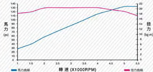
引擎性能曲線圖
